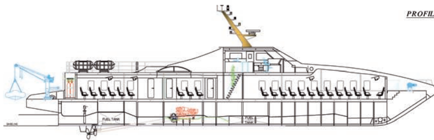
SEZIONE LONGITUDINALE
