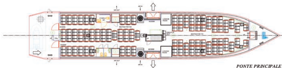
PONTE PRINCIPALE
