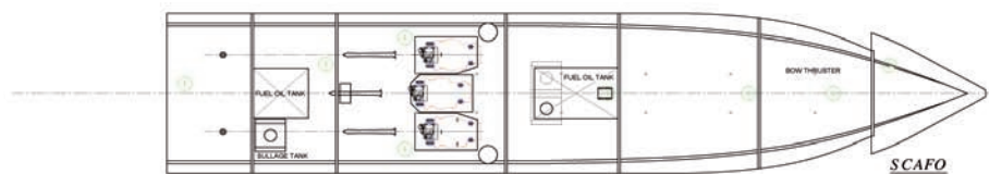
SCAFO
